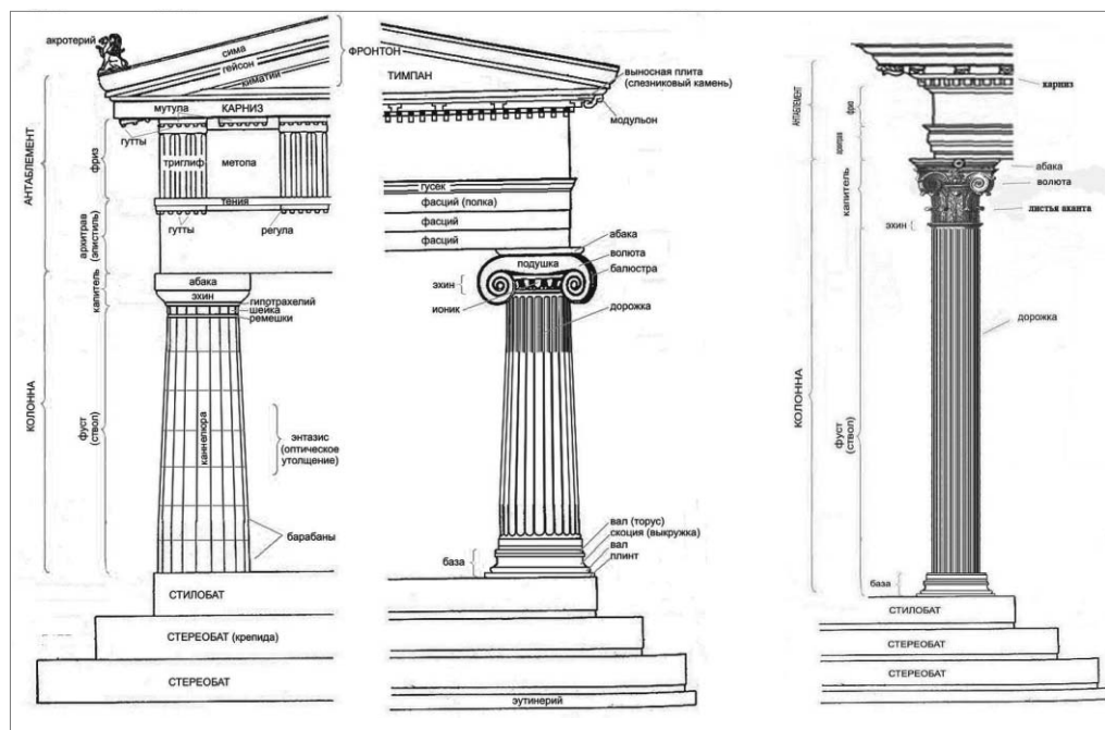
Типы греческих колонн: дорический ордер, ионический ордер, коринфский ордер
